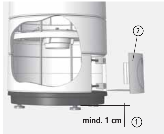
Abb. 2.1 Ausreichende Zuführung von Verbrennungsluft aus dem Raum
