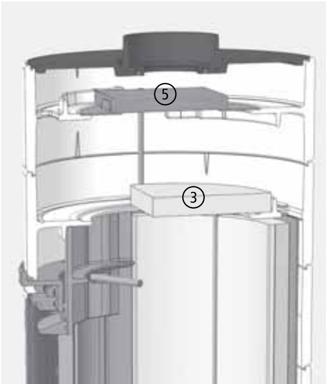
Abb. 3.4 Lage der Katalysatorplatten beim PEPPA tec, Schnittdarstellung
