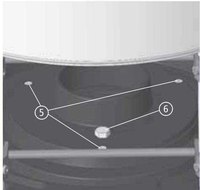
Abb. 3.31 Drehkonsolen-Oberteil montieren
