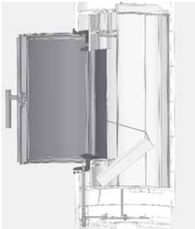
Abb. 4.31 Anheben des Bodensteins im Brennraum
