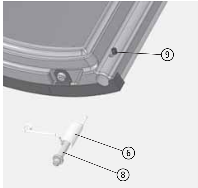
Abb. 3.14 Scharnierstift und Türfeder einsetzen
