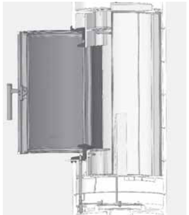
Abb. 4.32 Aufrichten des Bodensteins im Brennraum
