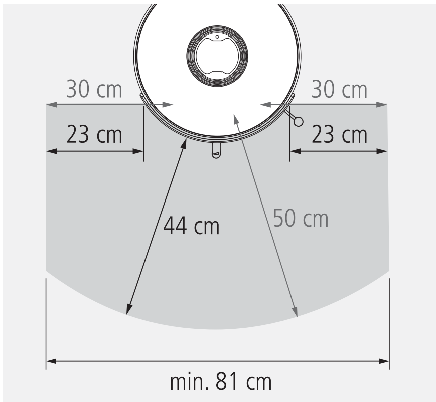
Abb. 1.2 Nicht brennbarer Belag vor der Feuerraumöffnung
