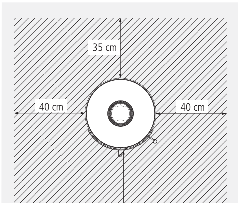
Abb. 1.1 Mindestabstände zu brennbaren Baustoffen oder Bauteilen
