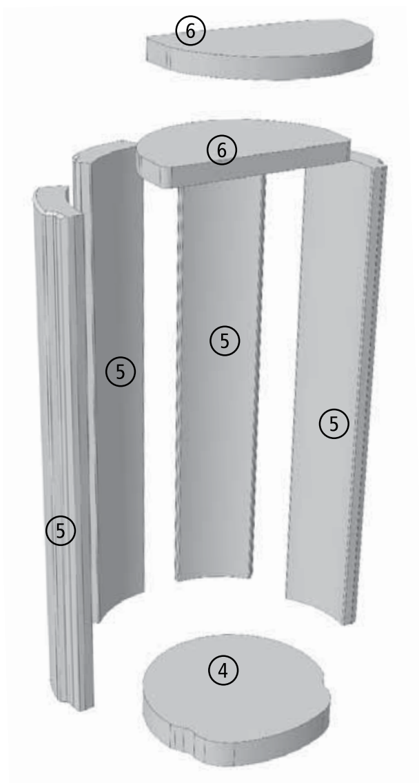
Abb. 5.1 Ersatzteilübersicht für PEPPA / PEPPA tec- Feuerraumauskleidung
