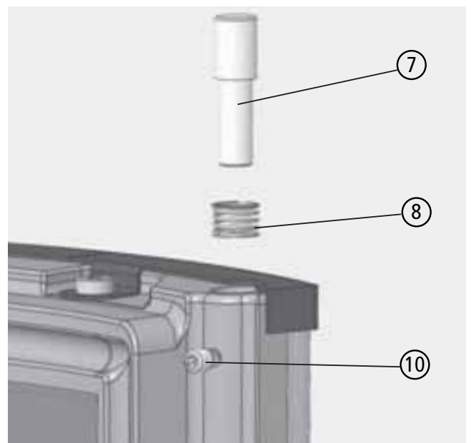
Abb. 3.9 oberer Scharnierstift mit Sicherungsfeder und Madenschraube
