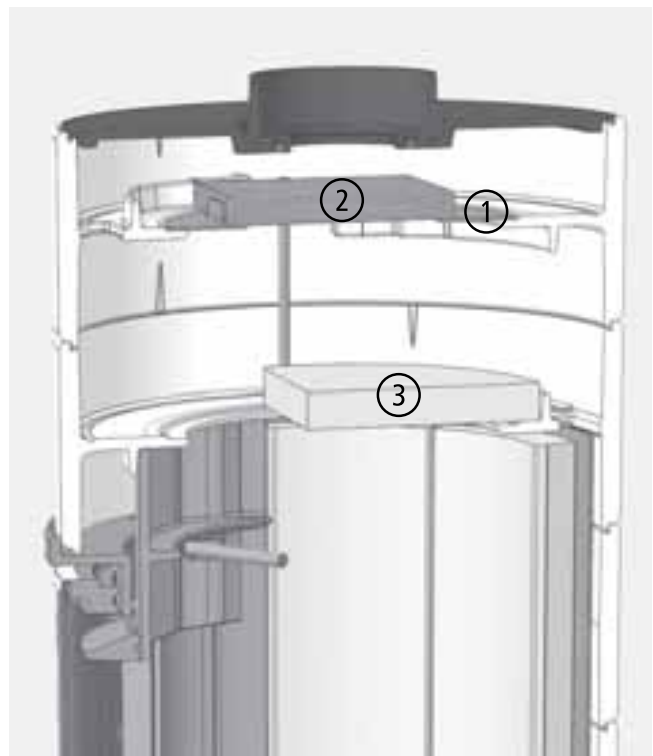
Abb. 3.21 Lage der Katalysator-Elemente beim PEPPA tec, Schnittdarstellung
