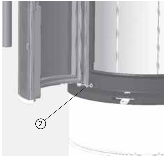
Abb. 3.7 Türfeder entspannen
