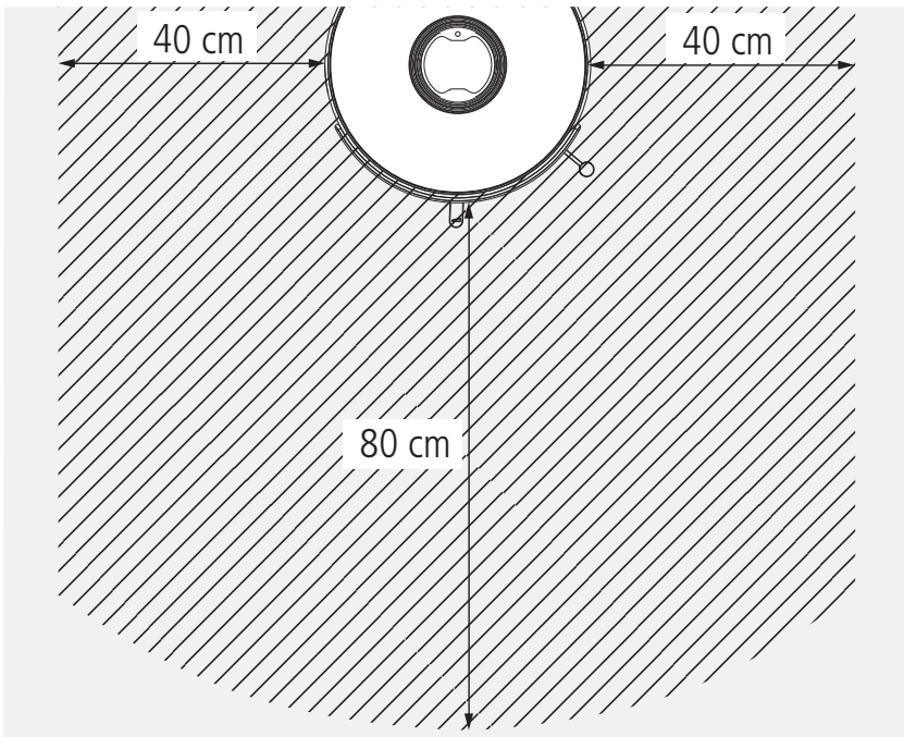
Abb. 1.3 Mindestabstände im Bereich der Sichtscheibe
