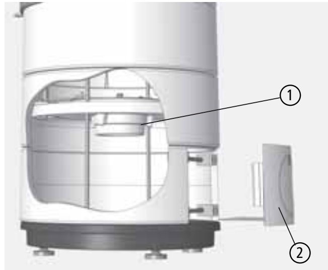
Abb. 3.1 Verbrennungsluftstutzen
