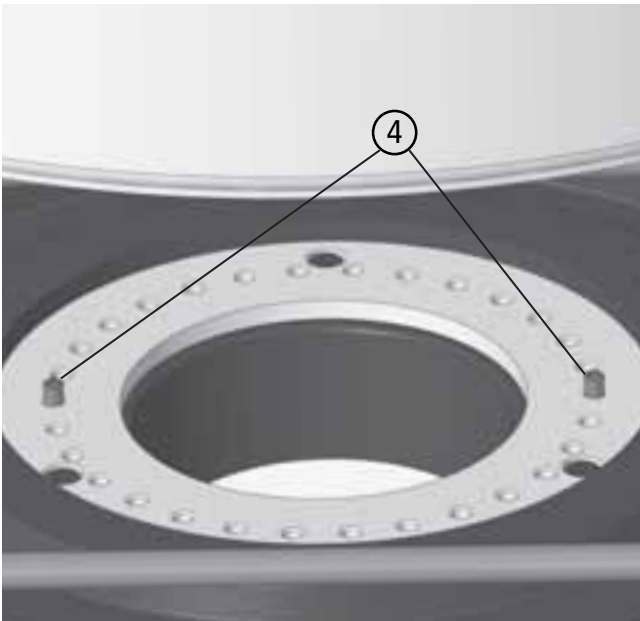
Abb. 3.30 Anschlag-Stifte, Einstellen des linken und rechten Endanschlags
