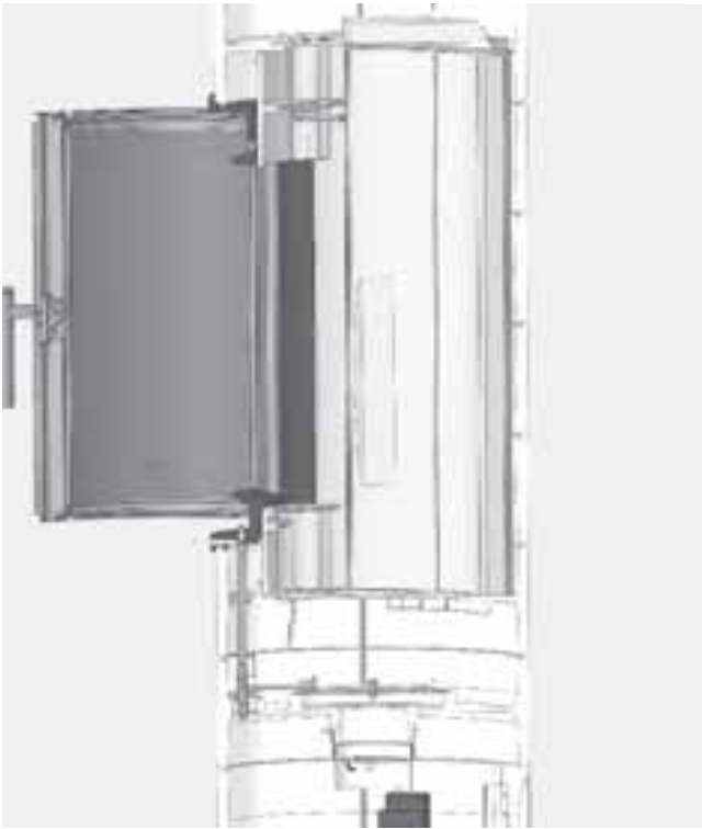
Abb. 4.33 Hochheben des Bodensteins im Brennraum
