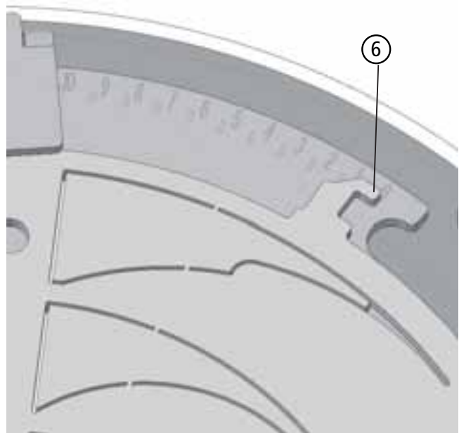
Abb. 3.40 Einstell-Skala des VSR auf dem Luftventil
