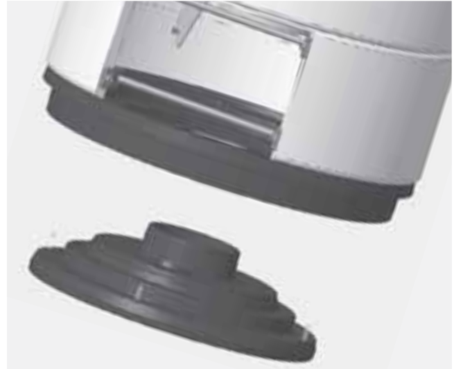
Abb. 3.27 Drehkonsole montieren
