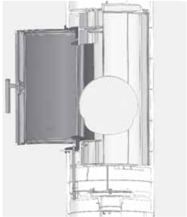
Abb. 4.35 Drehen des Bodensteins im Brennraum und Entnehmen
