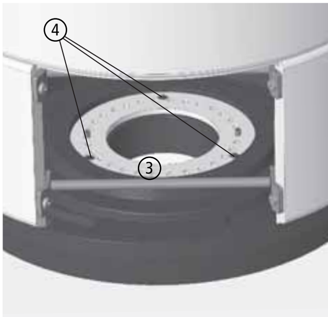
Abb. 3.33 Einstellscheibe für die seitlichen Anschläge ausbauen
