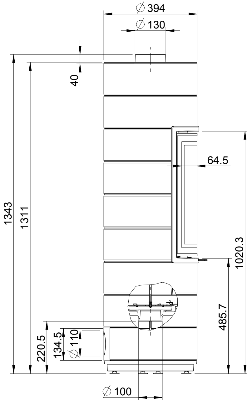
Abb. 3.35 Abgasanschluss, Maße
