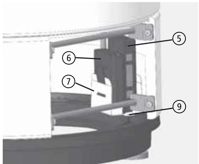
Abb. 3.20 Steuerung und Batteriegehäuse, elektronische Heizhilfe
