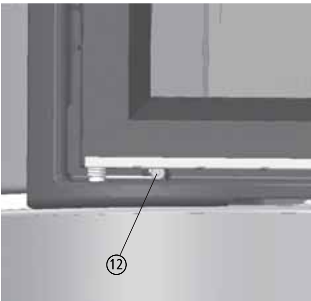
Abb. 3.15 Spannen der Türfeder
