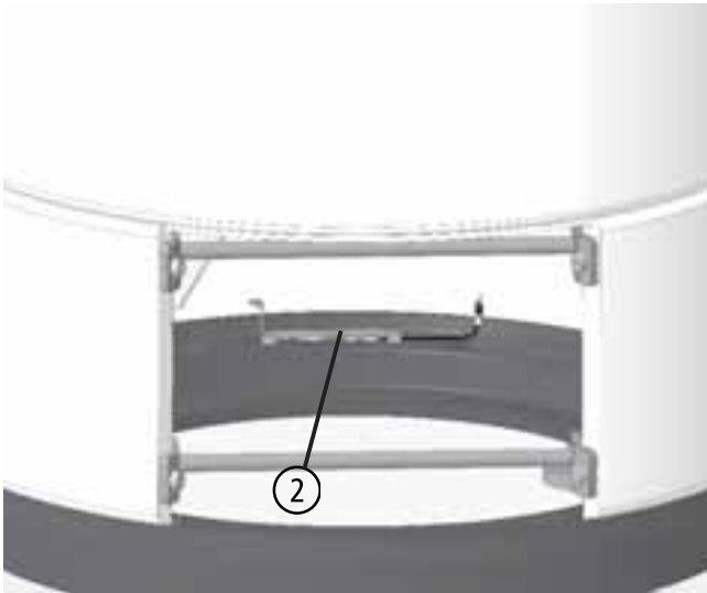
Abb. 3.18 LED-Element, elektronische Heizhilfe
