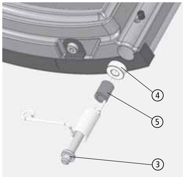
Abb. 3.13 unterer Scharnierstift mit Distanzhülsen
