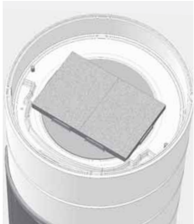
Abb. 3.5 Lage der Katalysatorplatten beim PEPPA tec, Blick von oben bei abgenommener Deckplatte
