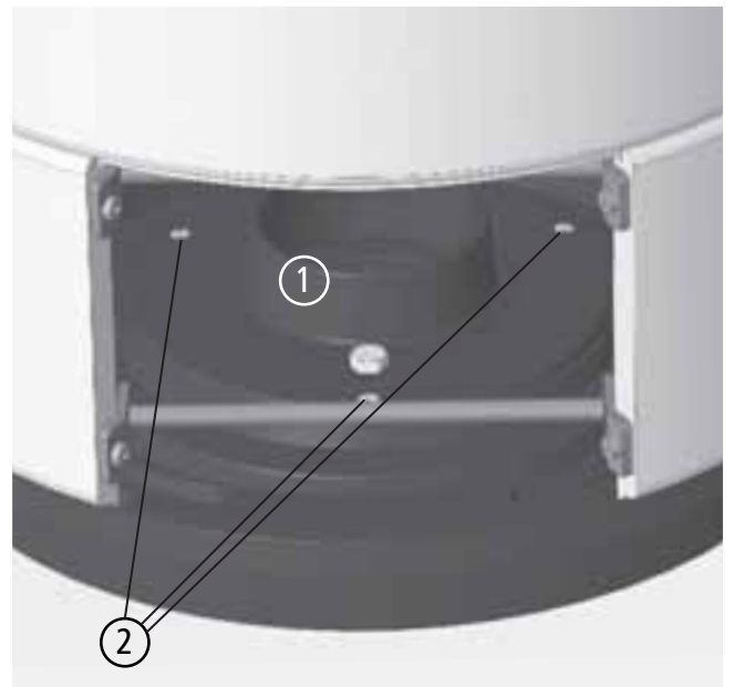
Abb. 3.32 Drehkonsolen-Oberteil abbauen
