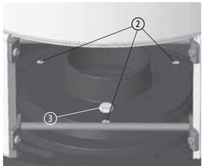
Abb. 3.28 Oberteil der Drehkonsole lösen
