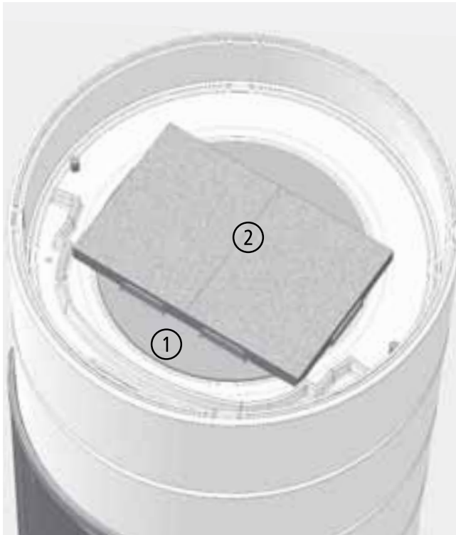
Abb. 3.22 Lage der Katalysator-Elemente beim PEPPA tec, Blick von oben bei abgenommener Deckplatte
