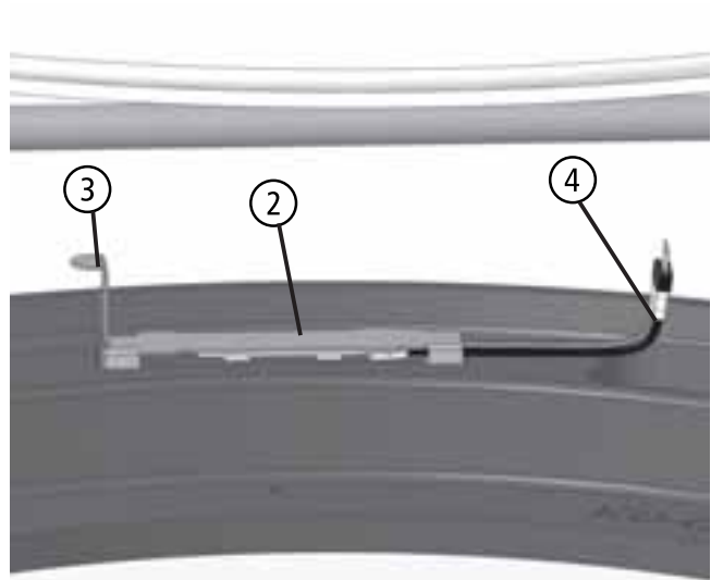
Abb. 3.19 LED-Element, elektronische Heizhilfe
