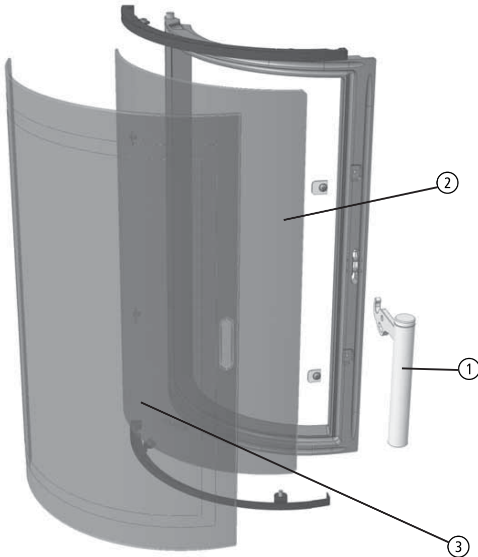
Abb. 5.2 Ersatzteilübersicht für PEPPA / PEPPA tec - Feuertür
